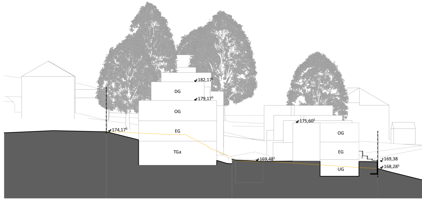
Schnitt 01
