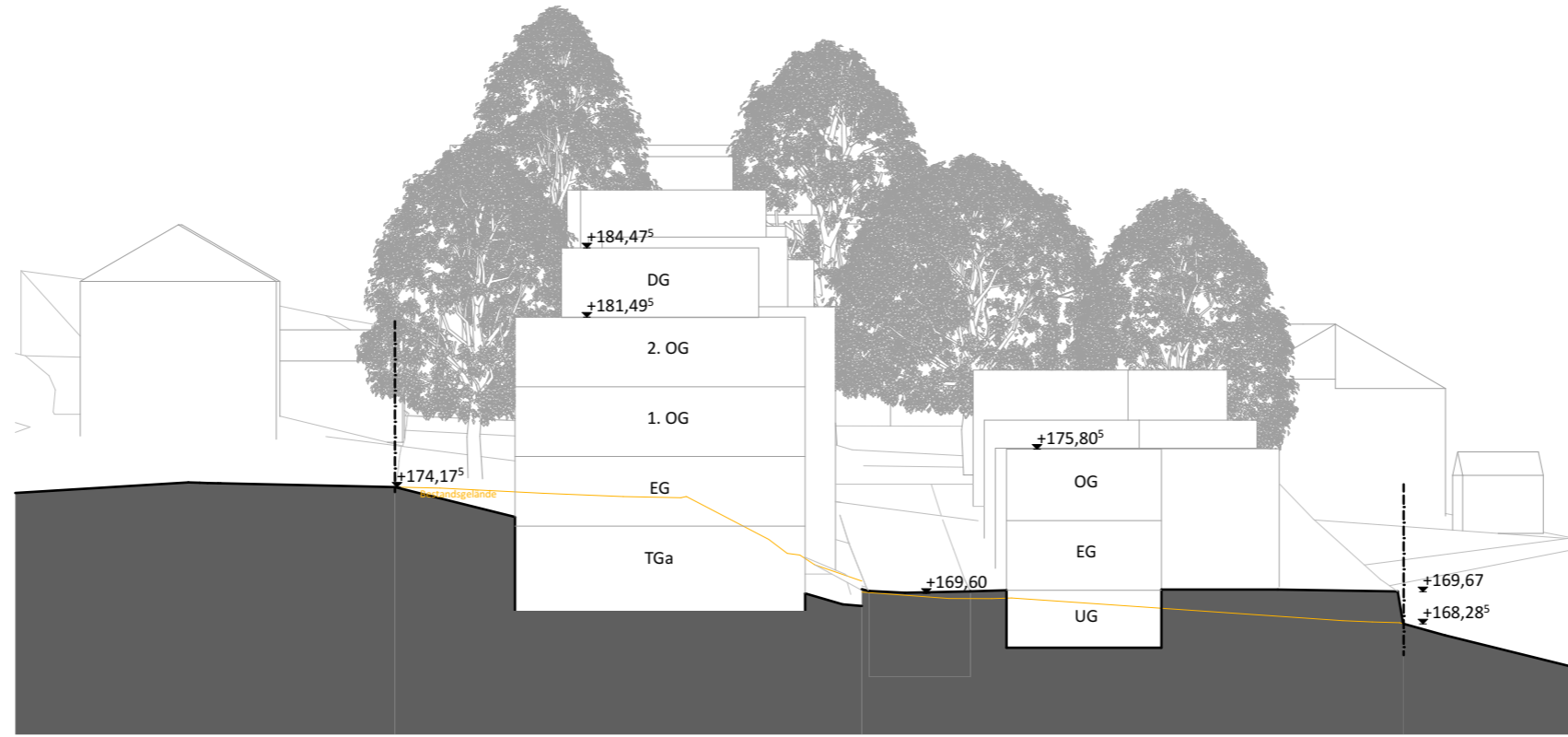
Schnitt 01
