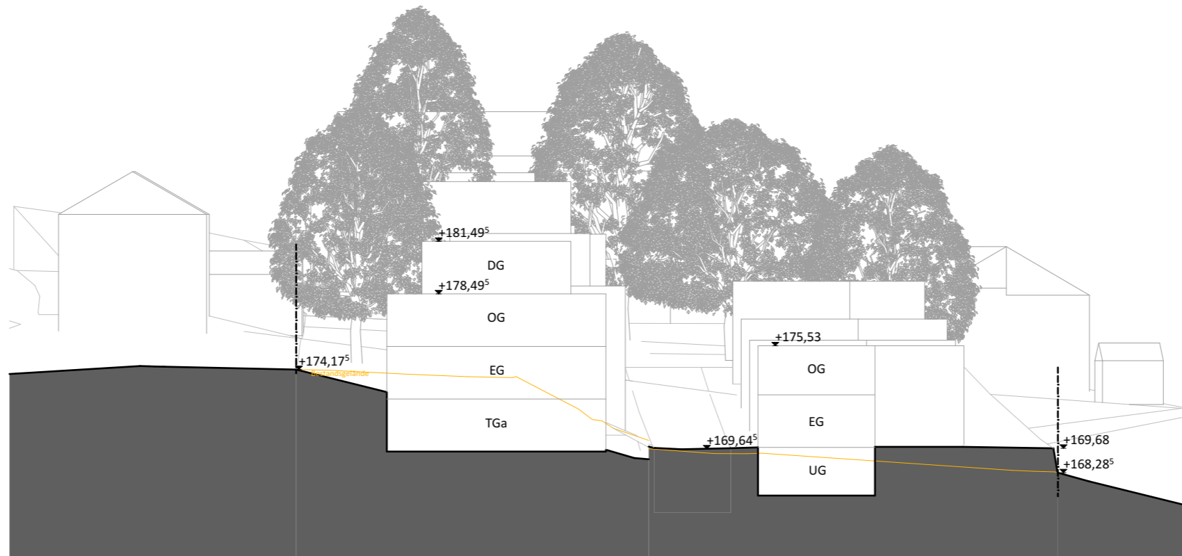
Schnitt 01
