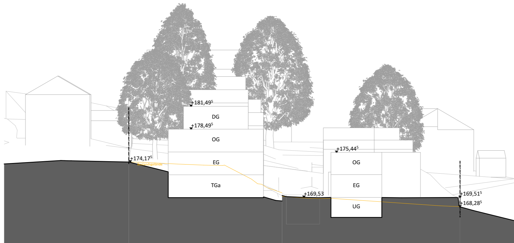
Schnitt 01
