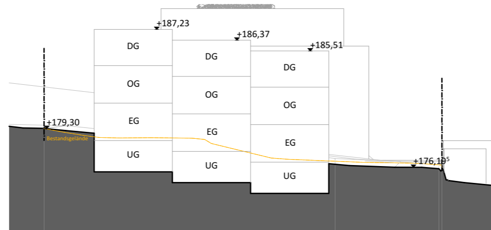
Schnitt 03
