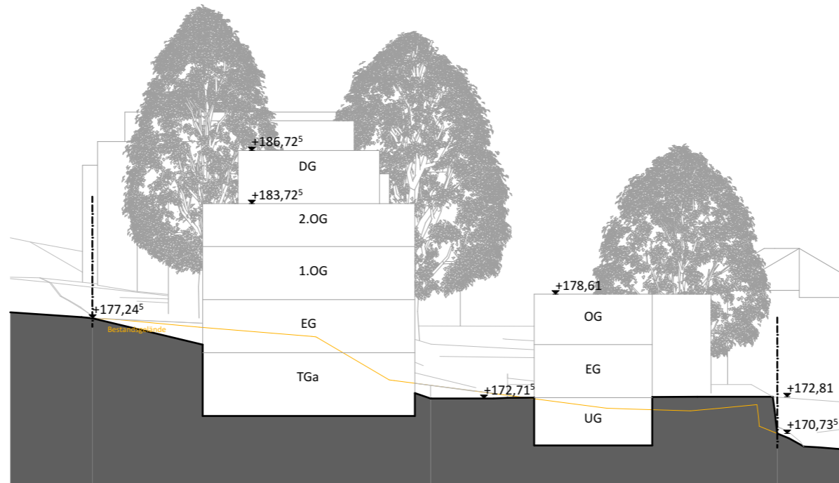
Schnitt 02
