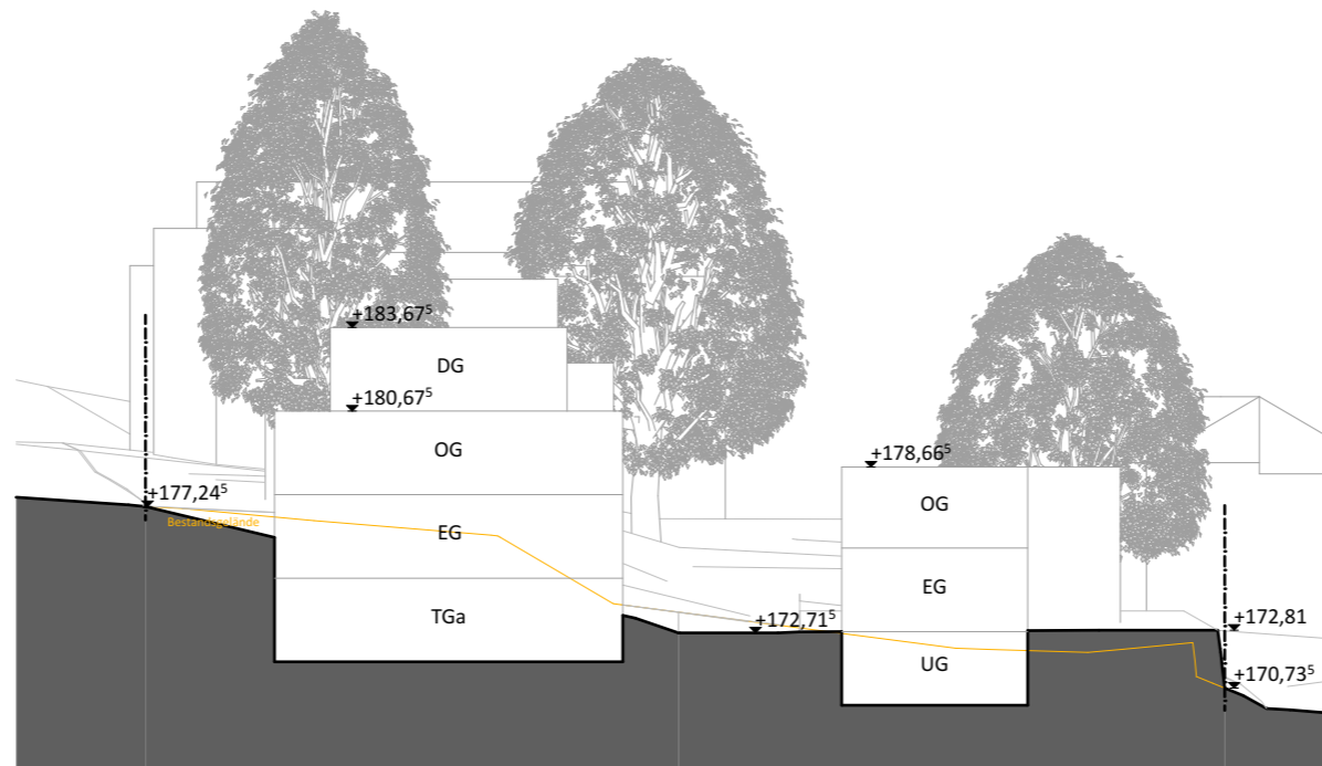
Schnitt 02
